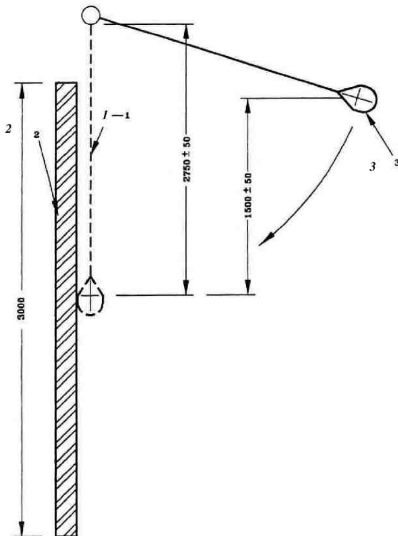
Рисунок 3 – Устройство для испытания на удар.
